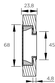
Sezione anta Door section
